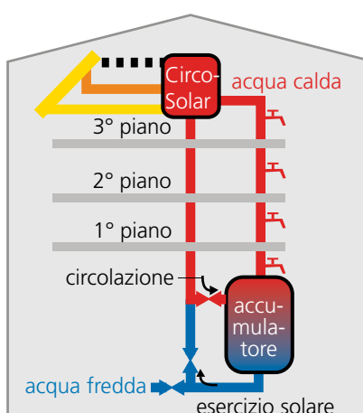
Sistema E: impianto CircoSolar Iniezione dell'acqua calda solare nella circolazione dell'acqua calda di una casa plurifamiliare. Non è necessario nessun accumulatore aggiuntivo; dipende dal dimensionamento delle condotte del circuito di circolazione dell'acqua calda; facile installazione sul tetto, brevi tratte di tubazione.
