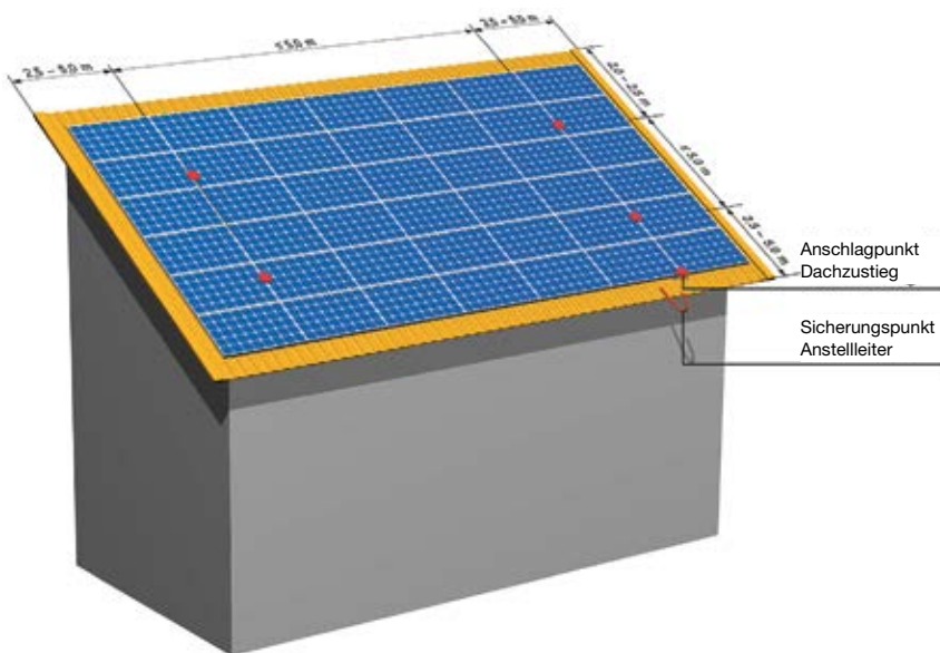
Bild 13 Beispiel einer Sicherung gegen Absturz mit Einzelanschlagnpunkten bei begehbaren Solarpanels (z.B. bei einem Pultdach)
