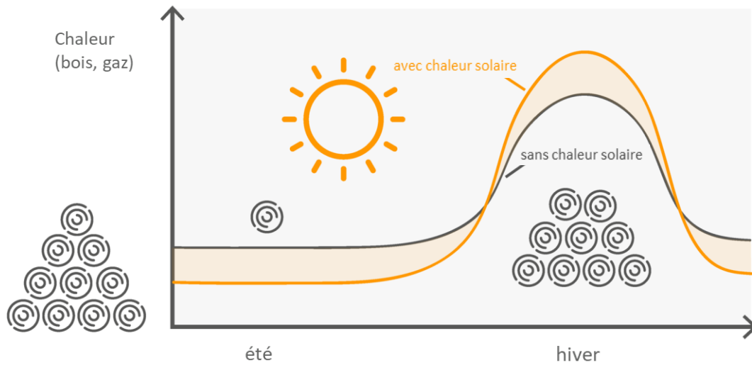
Fig. : Économie de bois, de gaz renouvelables et de déchets en été grâce à la chaleur solaire, et donc utilisation accrue de ces ressources en hiver.
