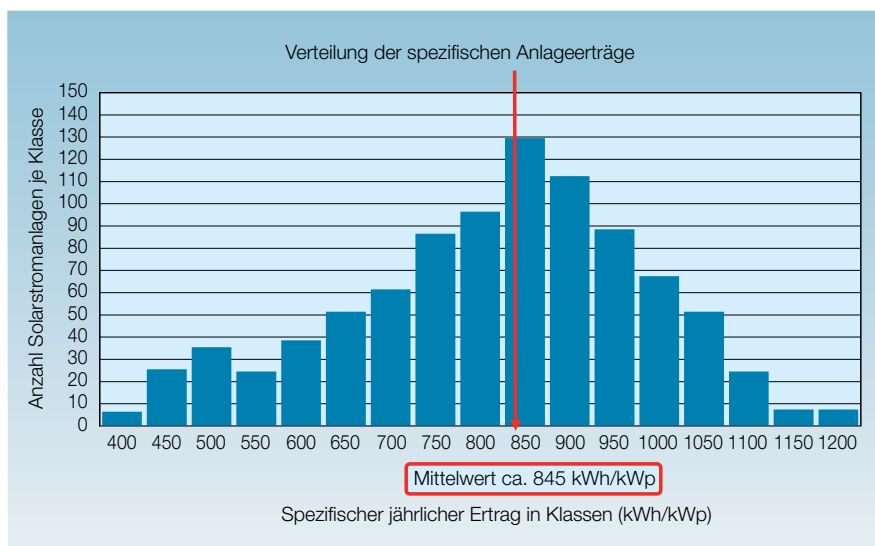
Bild 2: Der mittlere spezifische Jahresertrag der Solarstromanlagen im Jahre 2006 betrug gut 845 kWh/kWp. Er liegt unter anderem dank knapp 3,5% mehr Einstrahlung über dem langjährigen Mittel von 800 kWh/kWp.
