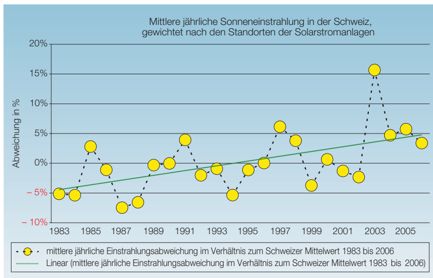
Bild 4: Verlauf der mittleren Einstrahlung in der Schweiz der letzten zwei Jahrzehnte. Die Sonneneinstrahlung lag im Jahr 2006 knapp 3,5% über dem langjährigen Mittel 1983–2005. Auffallend ist die stetige Aufwärtstendenz des Mittelwertes.
