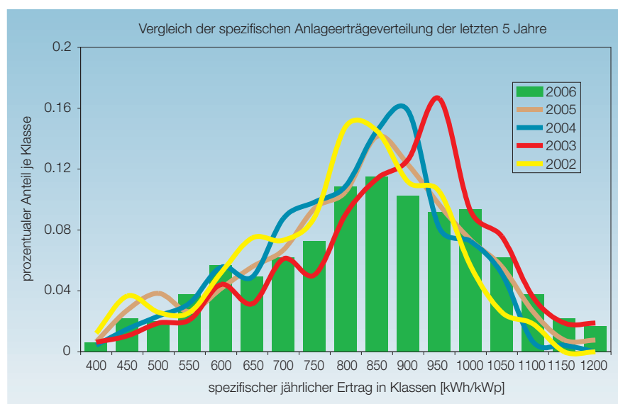
Bild 3: Spezifische Jahreserträge der Solarstromanlagen, aufgeteilt in 50-kWh/kWp-Klassen (Balkendiagramm), im Vergleich zu den Werten der Vorjahre (Linien).
