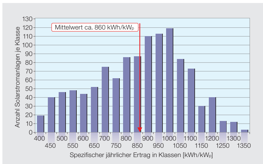
Bild 1 Der mittlere spezifische Jahresertrag der Solarstromanlagen im Jahre 2009 betrug gute 860 kWh/kW p . Er liegt unter anderem dank rund 3,0% mehr Sonneneinstrahlung über dem langjährigen Mittel von 820 kWh/kW p .
