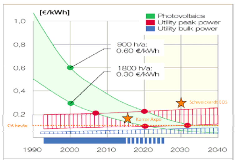
Grafico 1: Corrente solare verso la parità di rete in Europa. Fonte: EPIA, W. Hoffmann; completato
