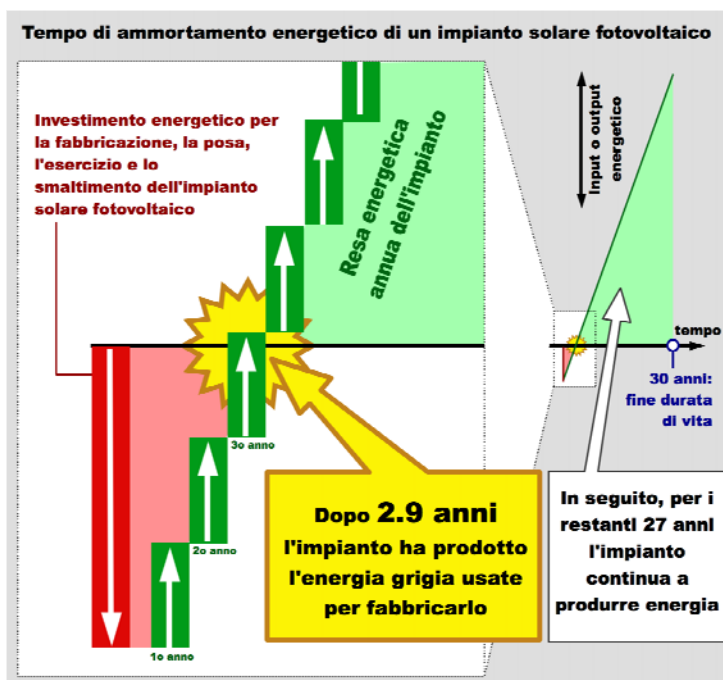
Grafico 3: Tempo di ammortamento energetico di un impianto fotovoltaico. Fonte: Swissolar / Doka
