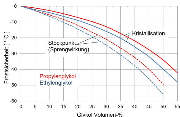
Abbildung 1: Frostsicherheit (°C) in Abhängigkeit des Glykol-Volumenanteils (vol.%) von propylen- und ethylen-basierten Wärmeträgern (Daten: Clariant)
